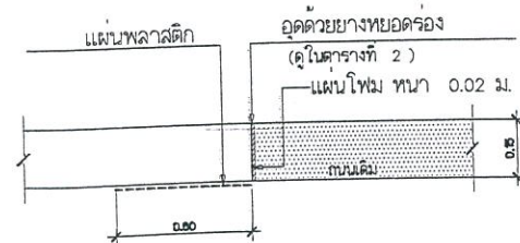
JOINT รอยต่อถนนเดิม Not To Scale
