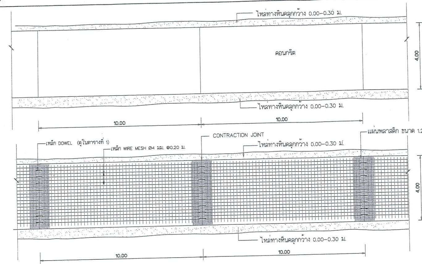
แปลนถนน คอนกรีตเสริมเหล็ก Not To Scale
